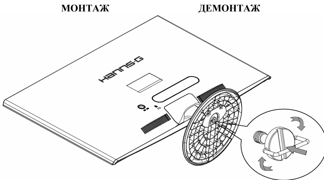
Фигура 1 Монтаж и демонтаж на основата
