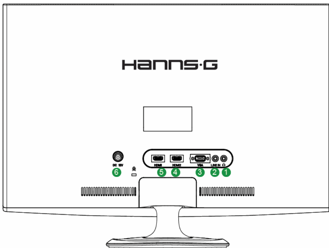
Фигура 2. Свързване на кабелите
