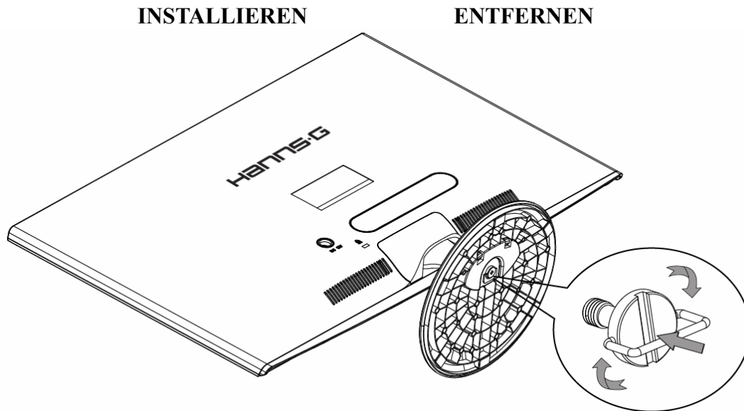
ABBILDUNG 1. INSTALLIEREN UND ENTFERNEN DES STÄNDERS
