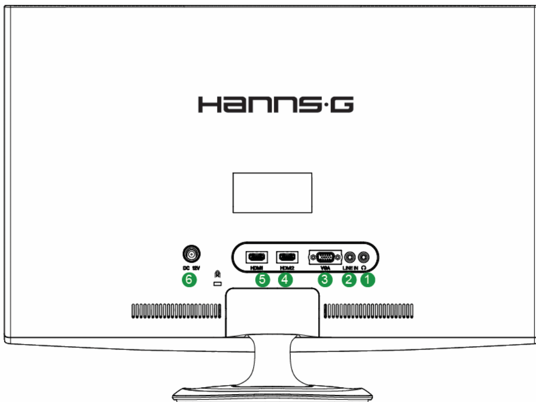
ABBILDUNG 2. ANSCHLISSEN AN EINEN PC
