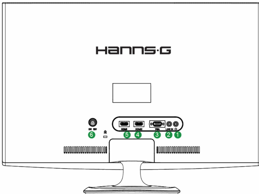
Figura 2. Conexión a un PC
