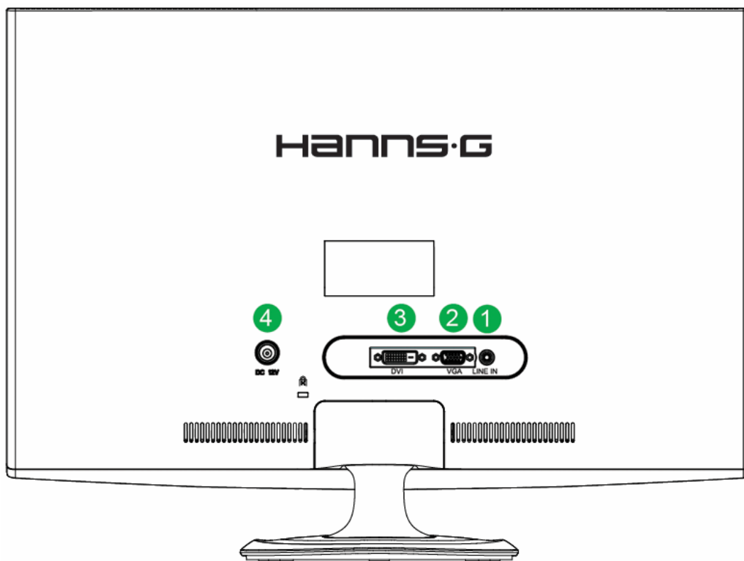
Figura 3. Conexión a un PC
