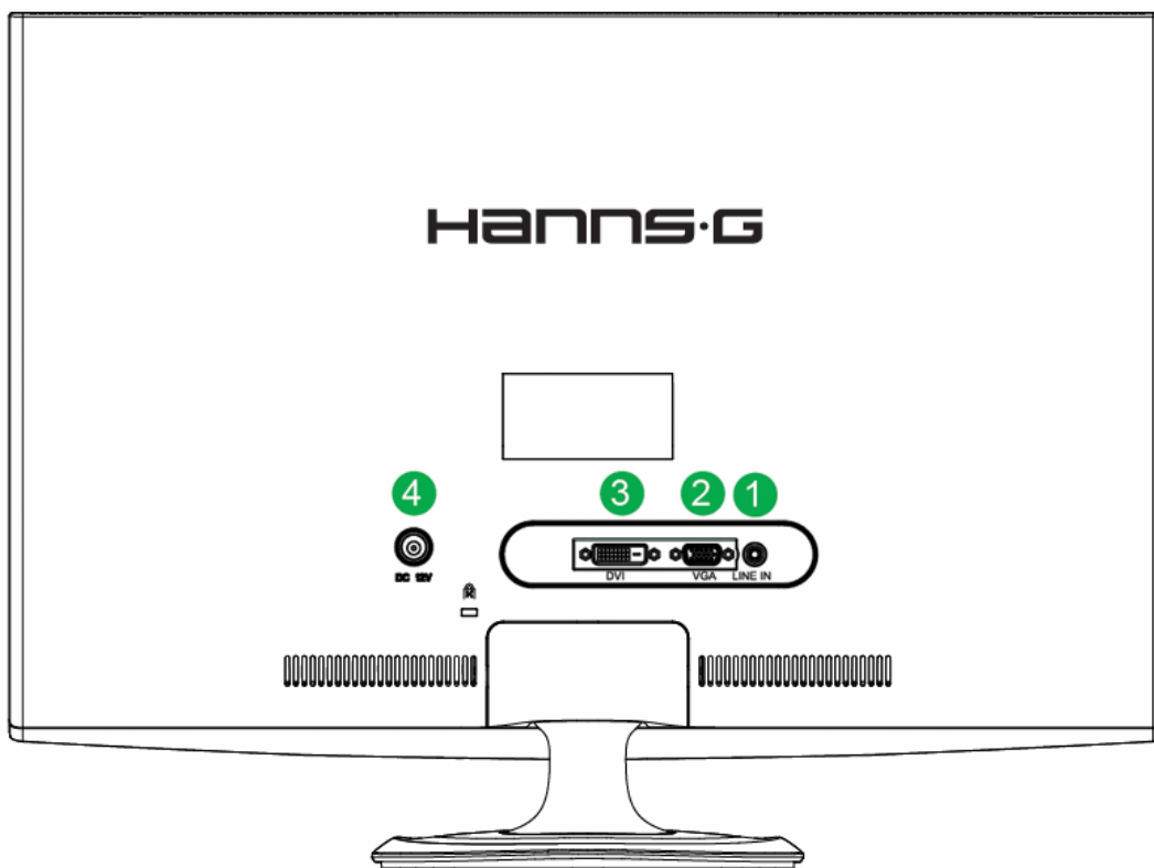
Εικόνα 3 Σύνδεση καλωδίων
